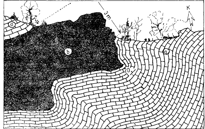
Şekil 3: Şekil 2 ile aynı.
