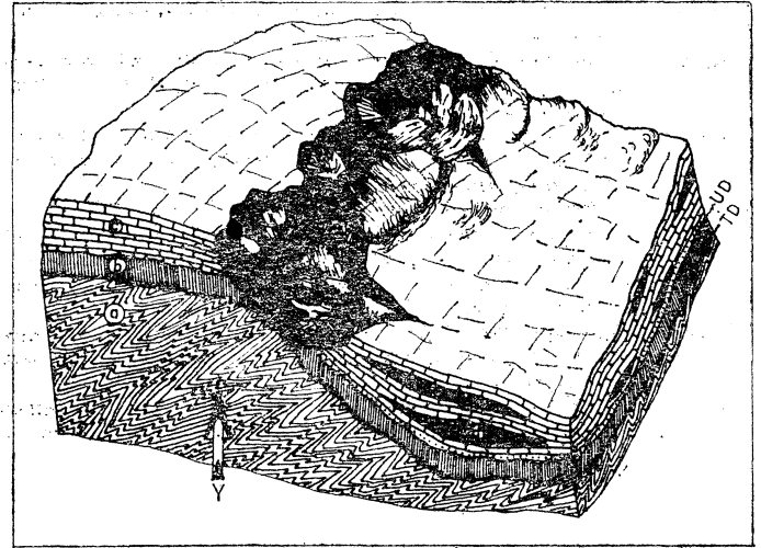
gekil 14: Çördük olistostromlarının oluşumunu gösteren blok diyagram, a) Permiyen yaflı başkalaşım kayaları (Tokat Masifi); TD: Tektonik dokaaak; b) Senomaniyen yağı ofiyolitli melanj; UD: Ağılı Uyumsuzluk; c) Kampaniyen-Maestrihtiyen yaşlı pelajik kireçtaşı (normal sedimanter istif); d) Çördük olistostromları; Y: Yüksleme.
