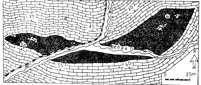
Şekil 2: Bileşenleri ofiyolitli melanjdan türemiş, Kampaniyen-Maestrihtiyen yaşlı bir olistostromun gömümü, a) Kampaniyen-Maestrihtiyen yaşlı pelajik kireçtaşı (normal sedimanter istif b) Ofiyolitli melanj olistostromu.
