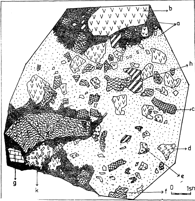
Sekil 8: Kampaniyen-Maestrihtiyen yağlı bir ofiyolitli melanj olistostromunun görünümü. a) Hamur; b) diyabaz ve metadiyabaz, c) Mermer, d) serpantin ve peridotit, e) granit ve diyorit, f) kuvars-klorit-albit gist, ve serizit-kuvars gist, g) kireçtaşı, h. radyolarit* k. diğer kayaç parçaları (bir el örneğinden çizilmiştir).
